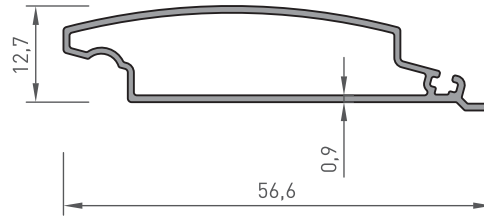
1058 GÜNEŞ KIRICI 0.315 kg / m
