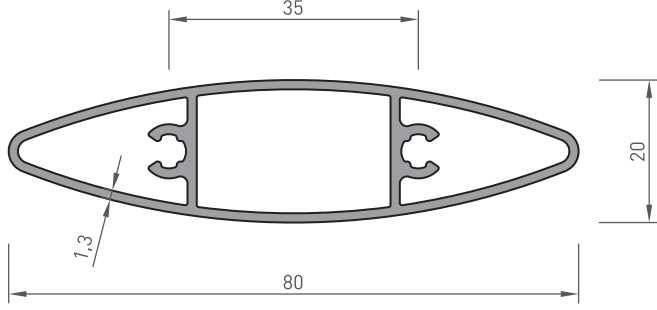
1000-170 GÜNEŞ KIRICI 0.820 kg/m
