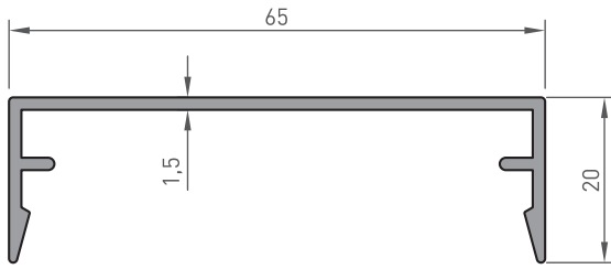
1000-126 20 LİK KAPAK 0.455 kg/m
