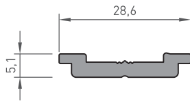
1000-349 TİJ 0.285 kg/m
