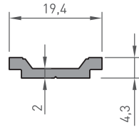
1042 TİJ ÇUBUĞU 0.135 kg/m
