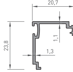
1000-204 CEPHE PROFİLİ 0.190 kg/m
