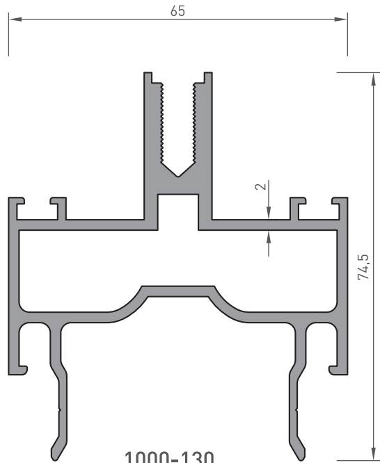
1000-130 YATAY TAŞIYICI MONTAJ PROFİLİ 1.900 kg/m
