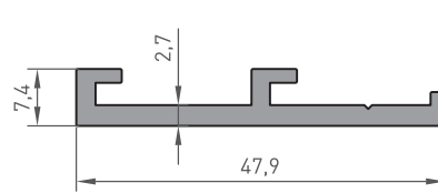
1000-277 CEPHE PROFİLİ 0.475 kg/m
