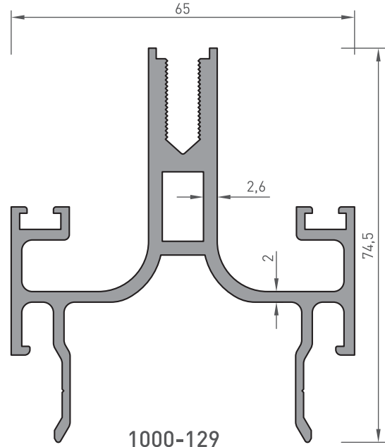
1000-129 DÜŞEY TAŞIYICI MONTAJ PROFİLİ 1.855 kg/m
