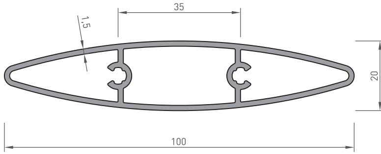
1000-172 GÜNEŞ KIRICI 1.045 kg/m
