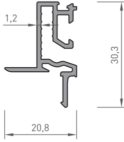
1000-206 KASET 0.305 kg/m
