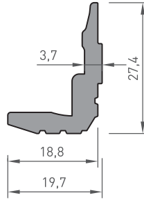
1000-207 CEPHE PROFİLİ 0.435 kg/m
