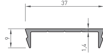
1000-246 PANEL ZEMİN ÜST KAPAK ÇITASI 0.205 kg/m
