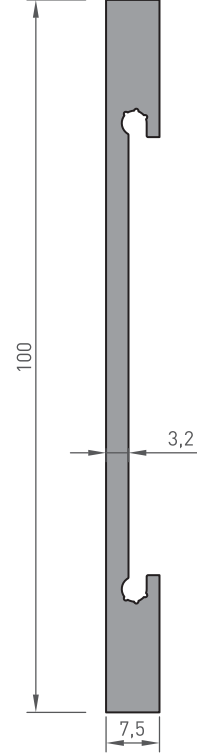
1000-185 GÜNEŞ KIRICI LAMA 1.265 kg/m
