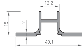
1028 KAPAMA PRF. 0.300 kg/m
