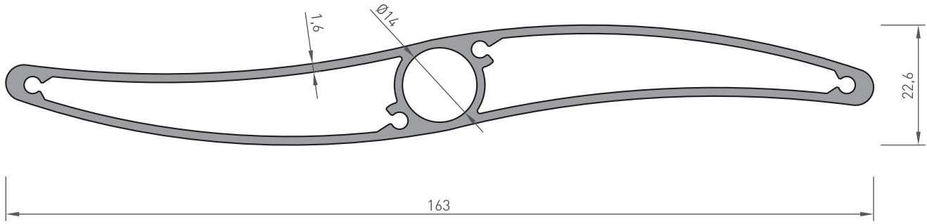
1000 -134 GÜNEŞ KIRICI 1.720 kg/m
