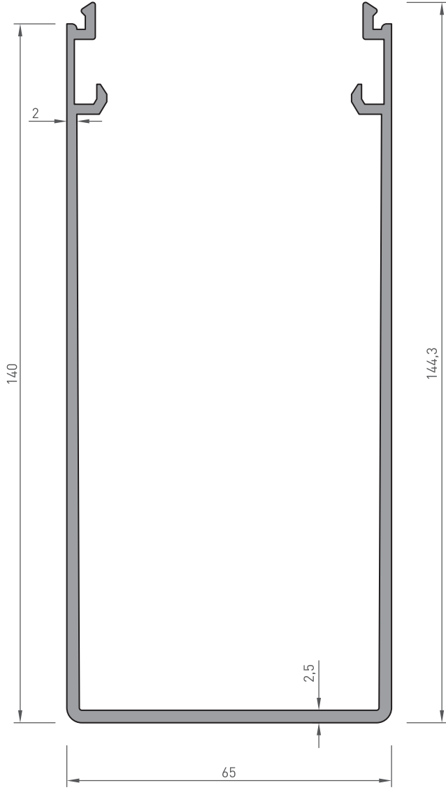
1000-123 140 LİK KASA 2.240 kg/m
