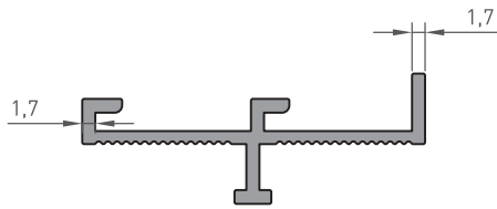
1000-276 CEPHE PROFİLİ 0.360 kg/m
