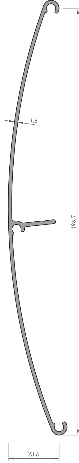
1000-304 GÜNEŞ KIRICI-YAPRAK 1.100 kg / m
