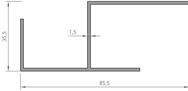
1000-323 DIŞ CEPHE PROFİLİ 0.710 kg/m
