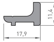
1039 CEPHE PRF. 0.240 kg/m
