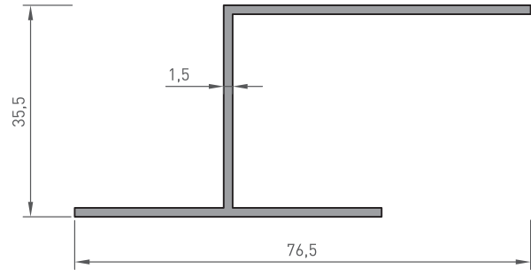
1000-324 DIŞ CEPHE PROFİLİ 0.570 kg/m
