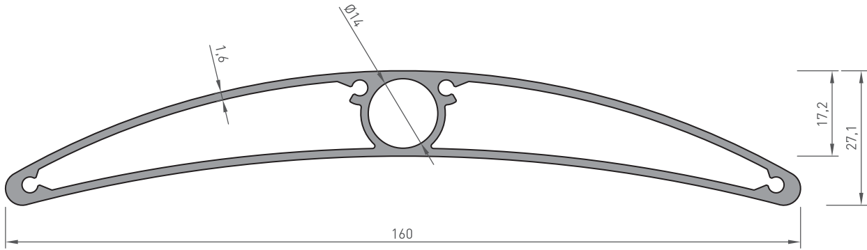
1000-174 160 GÜNEŞ KIRICI 1.725 kg/m
