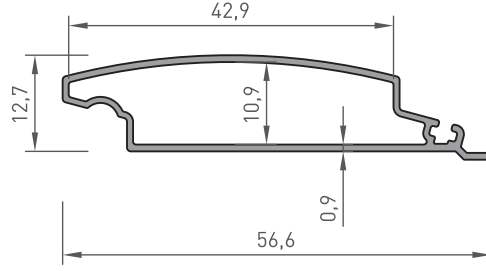
11-223 GÜNEŞ KIRICI 0.315 kg / m
