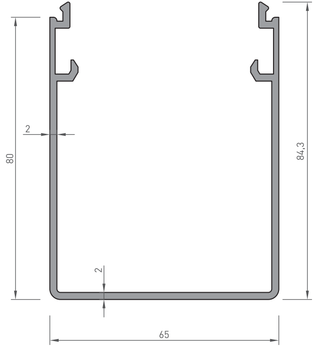
1000-124 80 LİK KASA 1.345 kg/m
