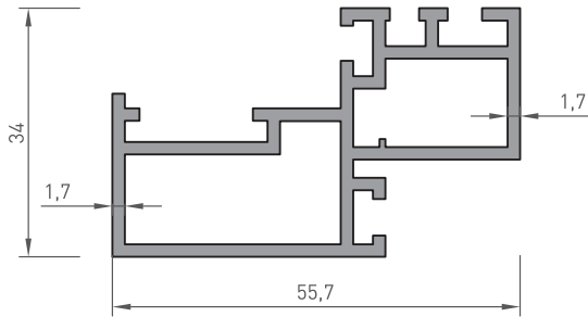
1000-322 KASET 1.020 kg/m
