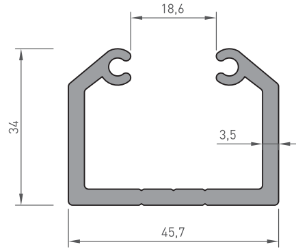
1076 CEPHE BAĞLANTI PROFİLİ 1.140 kg/m
