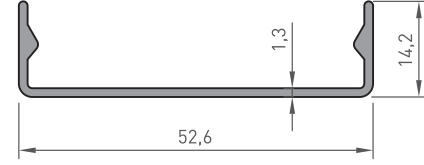
1000-331 15 LİK KAPAK 315 gr/m
