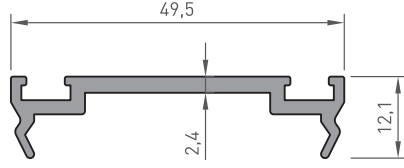
1000-330 KAPAK ALTI 0.455 kg/m
